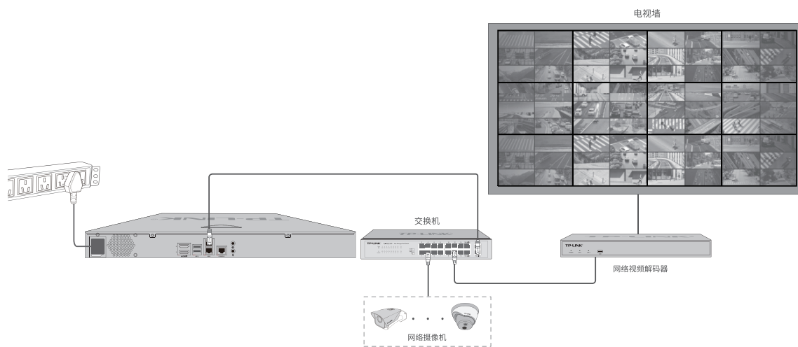
图3-1 设备连接示意图
