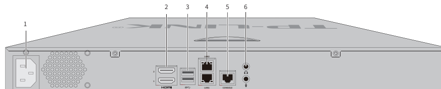
图1-3 TL-TUMS1500后面板示意图
